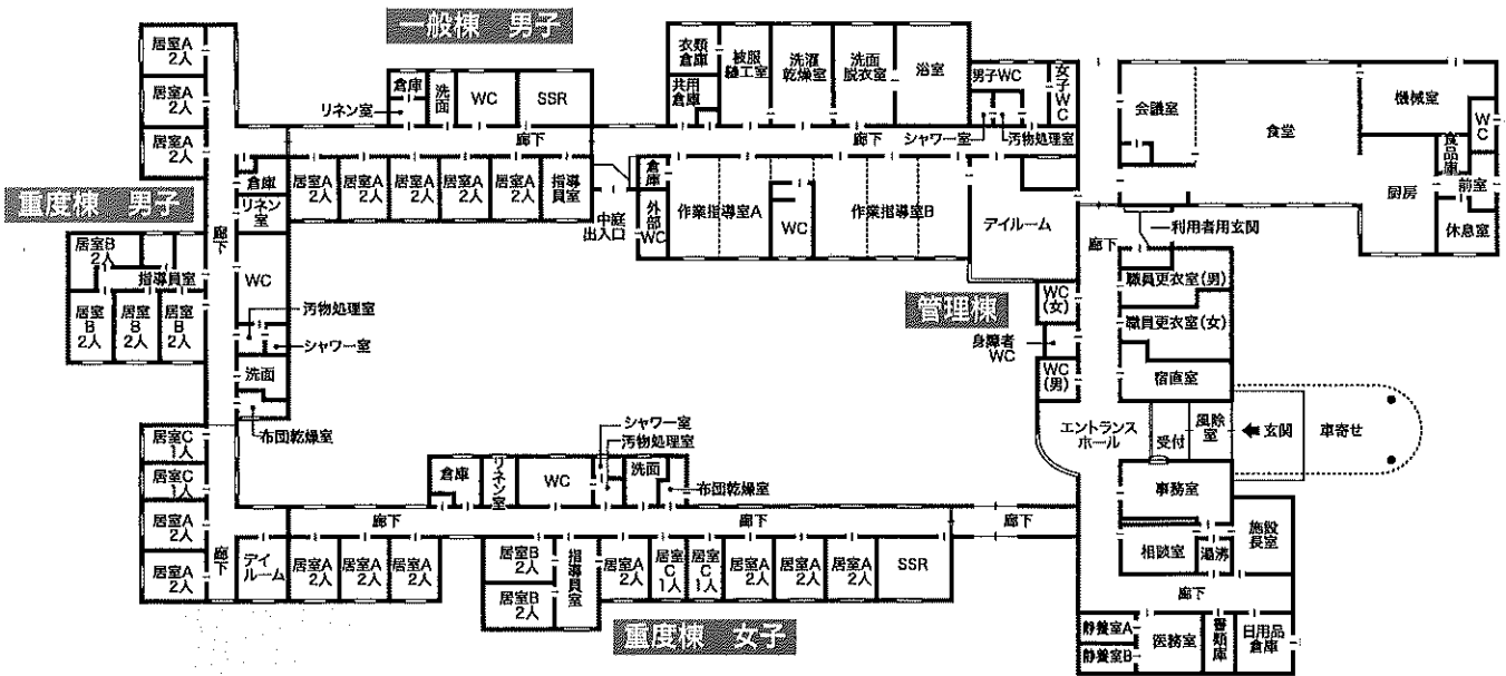
平面図
