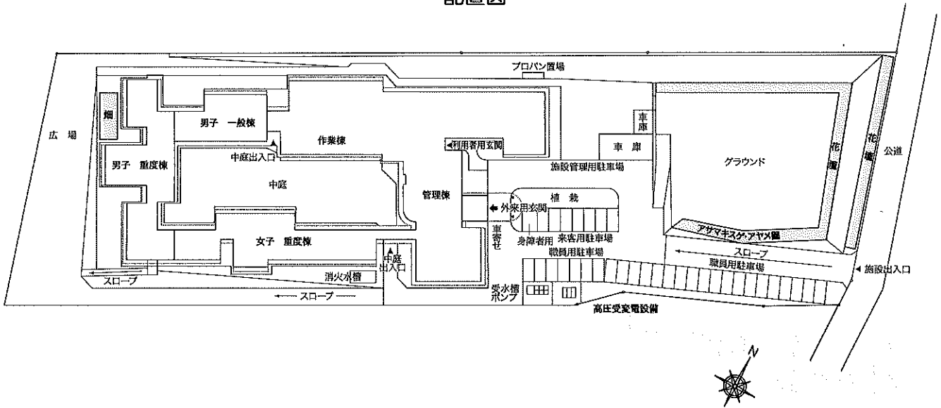
配置図
